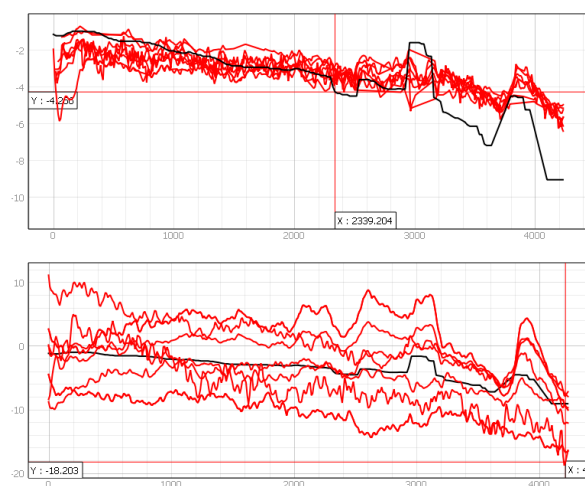
Figura 3. Na imagem do topo está a comparação entre os dados do ICESAT-2 (linha preta) e os resultados do modelo NN (linhas vermelhas). Em baixo, as linhas de cor vermelha representam os perfis do modelo de Stumpf em comparação com o mesmo perfil ICESAT-2. Nas duas imagens, o eixo dos xx representa a distância ao longo do perfil (m) e eixo dos yy representa a profundidade (m).
