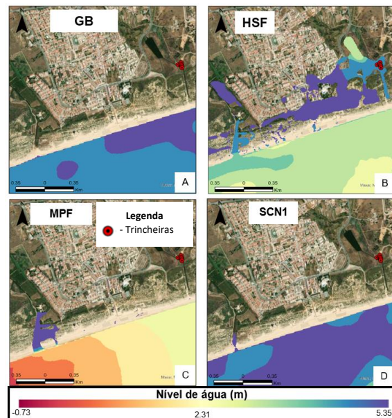
Figura 5. Resultados da modelação hidrodinâmica das fontes sísmicas: GB (A), HSF (B), MPF (C) e SCN1 (D).
