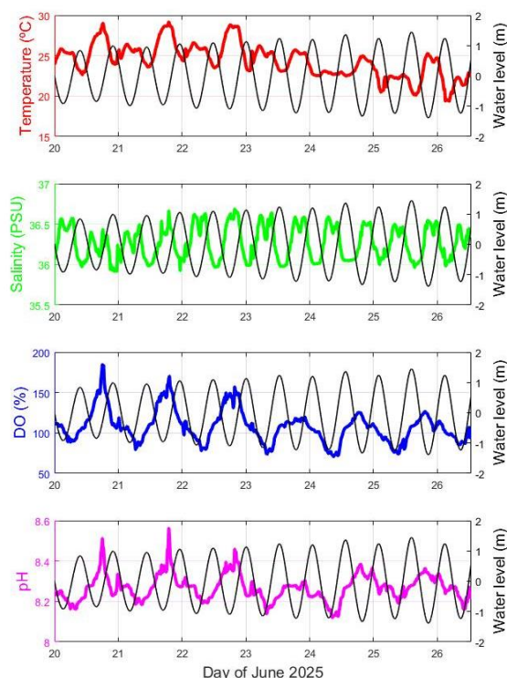
Figura 3. Variação da temperatura da água, salinidade, pH e percentagem de saturação de oxigénio dissolvido pela sonda multiparamétrica NKE, instalada na boia oceanográfica fundada na Praia dos Cavacos, Canal de Marim, na Ria Formosa, no âmbito do projeto CONNECT*, no período semanal de 20 a 27 de junho.
