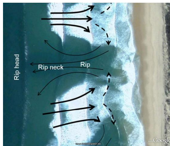
Figura 1.- Esquema tipo de la formación de las corrientes de resaca. Fuente: Mike Miloshs (2011).
