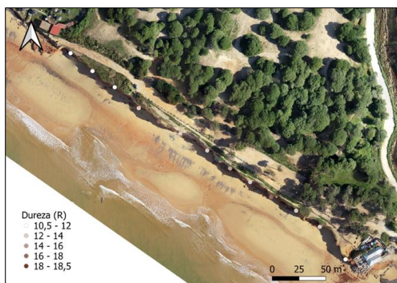
Figura 4. Variação dos valores de dureza da face da arriba medidos com o martelo de Schmidt.
