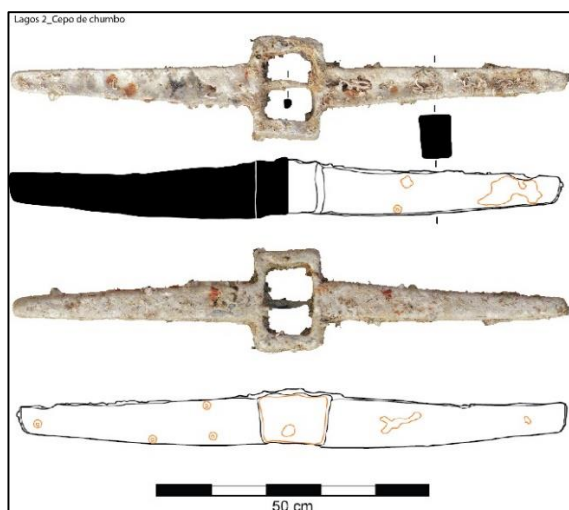
Figura 1. Lagos 2 – Cepo de chumbo de âncora romana (CNS 37377) recuperado em Março de 2024, pelo CNANS/PCIP.
