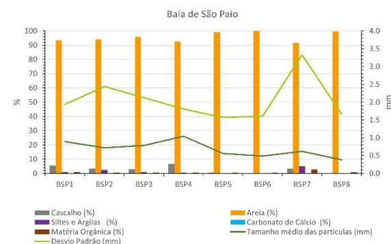
Figura 2. Resultados da análise textural (percentagens em cascalho, areia, e siltes e argilas), dos teores em carbonato de cálcio e matéria orgânica, e dos parâmetros estatísticos (média e desvio padrão), das amostras da Baía de São Paio.
