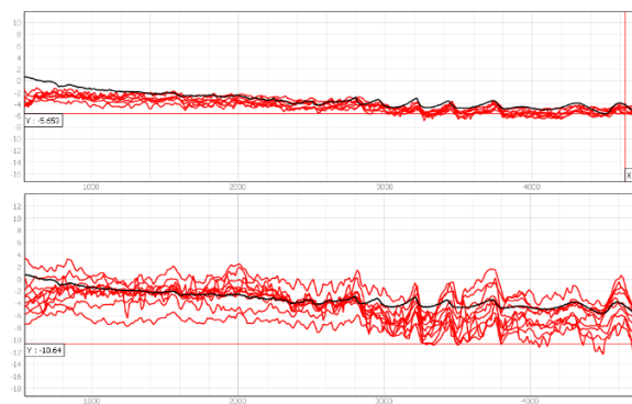
Figura 2. Na imagem em cima, estão representados a preto o perfil de feixe simples da APA, e a vermelho os perfis obtidos com o modelo NN. Em baixo, as linhas de cor vermelha representam os dados do modelo de Stumpf , ao longo do mesmo perfil da APA (a preto). Nas duas imagens, o eixo dos xx representa a distância ao longo do perfil (m) e eixo dos yy representa a profundidade (m).
