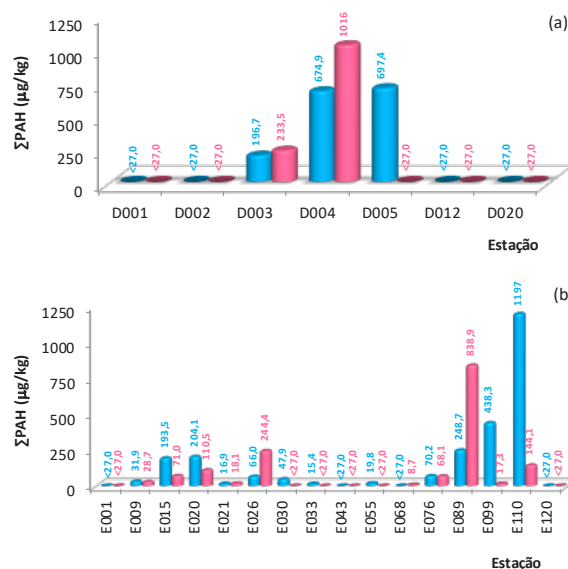
Figura 2. Teores totais de PAH parentais determinados ( \Sigma PAH; <27,0 \mu\text{g/kg} – limite de quantificação) nos sedimentos recolhidos nas duas épocas de amostragem nas áreas (a) D e (b) E. ● Out2018; ● Out2019.
