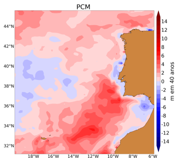
Figura 2. Tendências no Verão, junho-julho-agosto (JJA), de 1981 a 2020 calculadas pelo método de Theil-Sen da profundidade da camada de mistura (PCM) obtida da reanálise SODA3.2.15.
