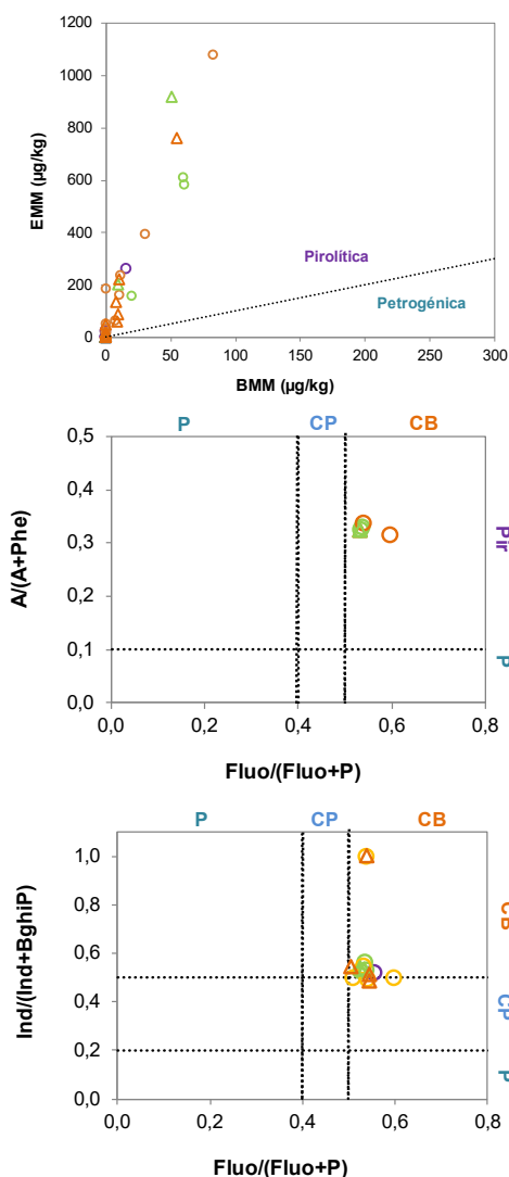
Figura 3. Teores de PAH, razões de diagnóstico e faixas limitrofes (Tobiszewski e Namieśnik, 2012) para classificação da origem de PAH (EMM – PAH de elevada massa molecular, BMM – PAH de baixa massa molecular, A – Antraceno, Phe – Fenantreno, Ind – Indeno(1,2,3-cd)pireno, BghiP – Benzo(g,h,i)perileno, P – Petrogénica, CP – Combustão de combustíveis fósseis, CB – Combustão de biomassa, Pir – Pirolítica): ○ Área A (Out2018), △ Área A (Maio2020), ○ Área B (Mar2019), △ Área B (Maio2020), ○ Área C (Mar2019), △ Área C (Out2019), ○ Área D (Out2018), △ Área D (Out2019), ○ Área E (Out2018) e △ Área E (Out2019). Ausência de dados nos gráficos aponta para o facto de pelo menos uma das razões de diagnóstico ou teor de PAH não ter sido determinada em consequência de existir teores inferiores ao limite de quantificação do método.
