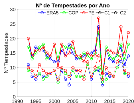
Figura 3. Número de tempestades por ano, considerando os critérios C1 e C2, para as diferentes bases de dados.
