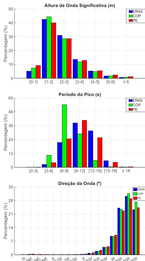
Figura 2. Distribuições da altura significativa das ondas, período de pico e direção média, para as diferentes bases de dados (1993 a 2021).
