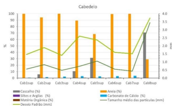
Figura 3. Resultados da análise textural (percentagens em cascalho, areia, e siltes e argilas), dos teores em carbonato de cálcio e matéria orgânica, e dos parâmetros estatísticos (média e desvio padrão), das amostras do Cabedelo.
